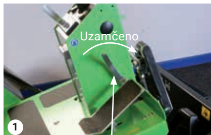
Přepravní zámek
